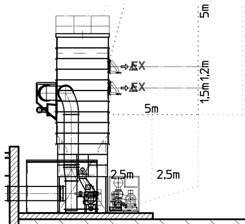
Coupe de profil
