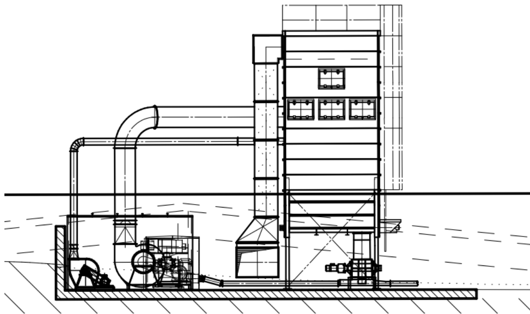
Coupe de face
